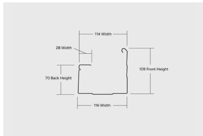
EASILINE® DOMESTIC (WA)
