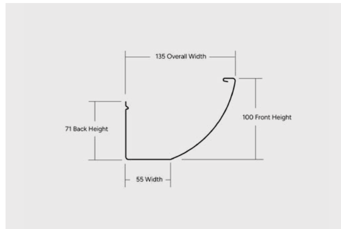
QUARTER ROUND (WA)
