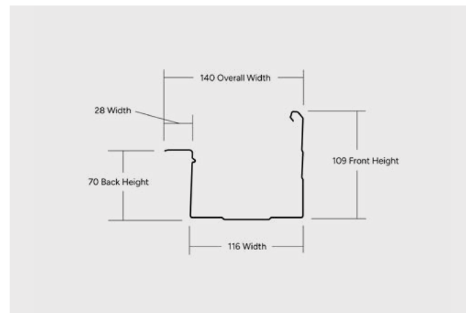
EASILINE® PATIO (WA)
