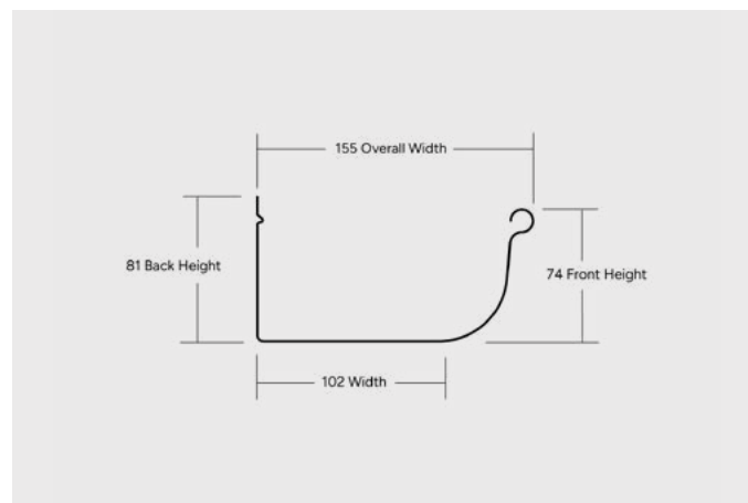
QUAD 150 (QLD) LO FRONT
